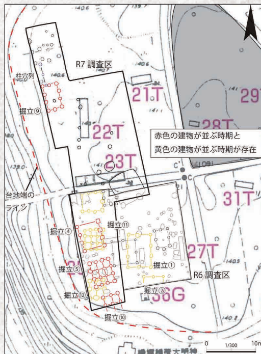
▲建物の配置
