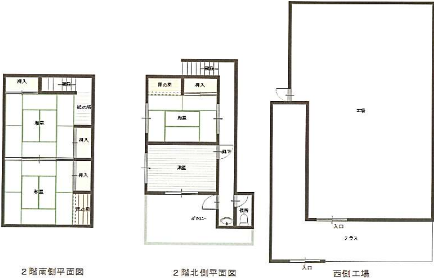
2階・工場倉庫 平面図
