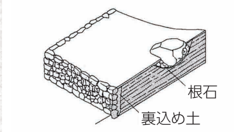
▲基壇イメージ図(文化庁2013より引用)
