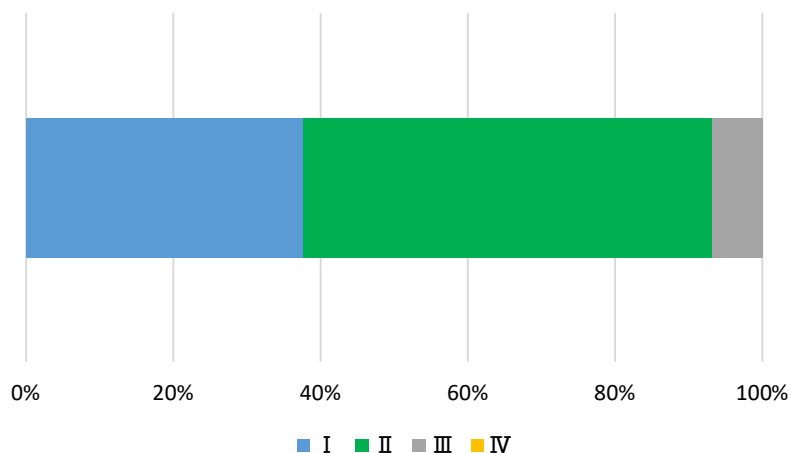
点検結果の状況(道路橋)
